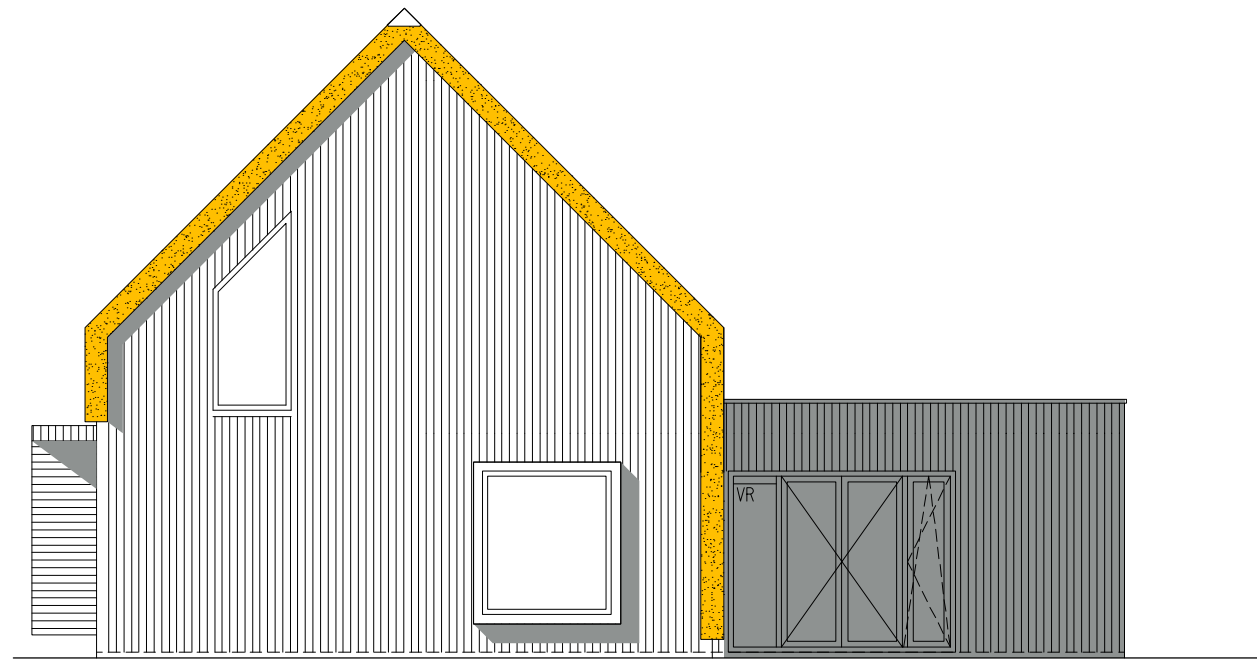
KOPGEVEL
