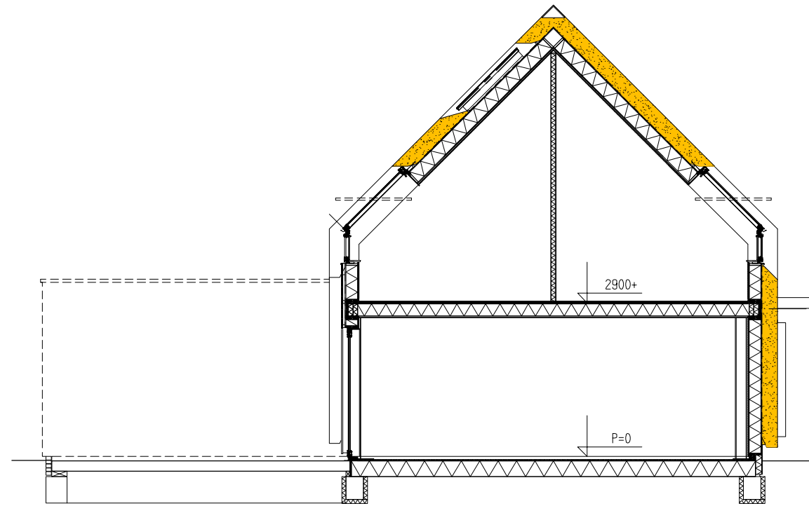
PRINCIPE DOORSNEDE 2
