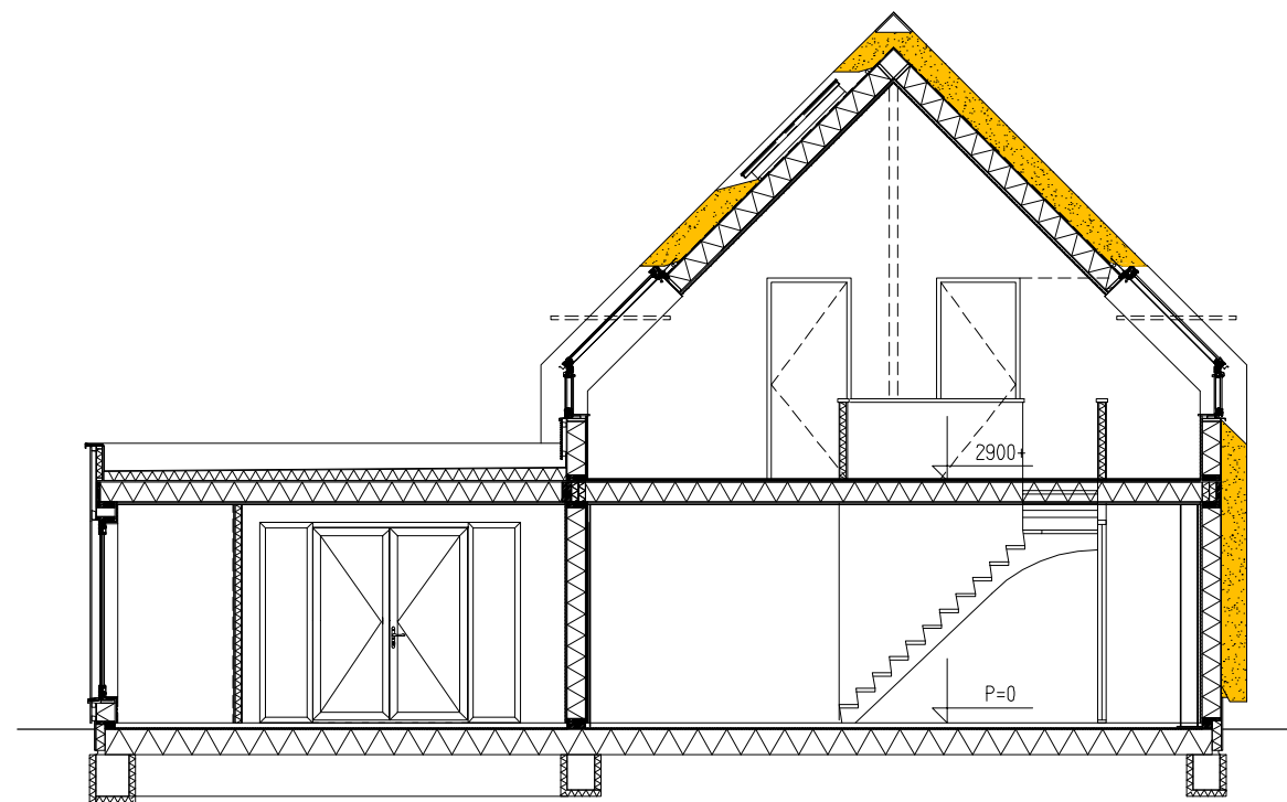
PRINCIPE DOORSNEDE 2
