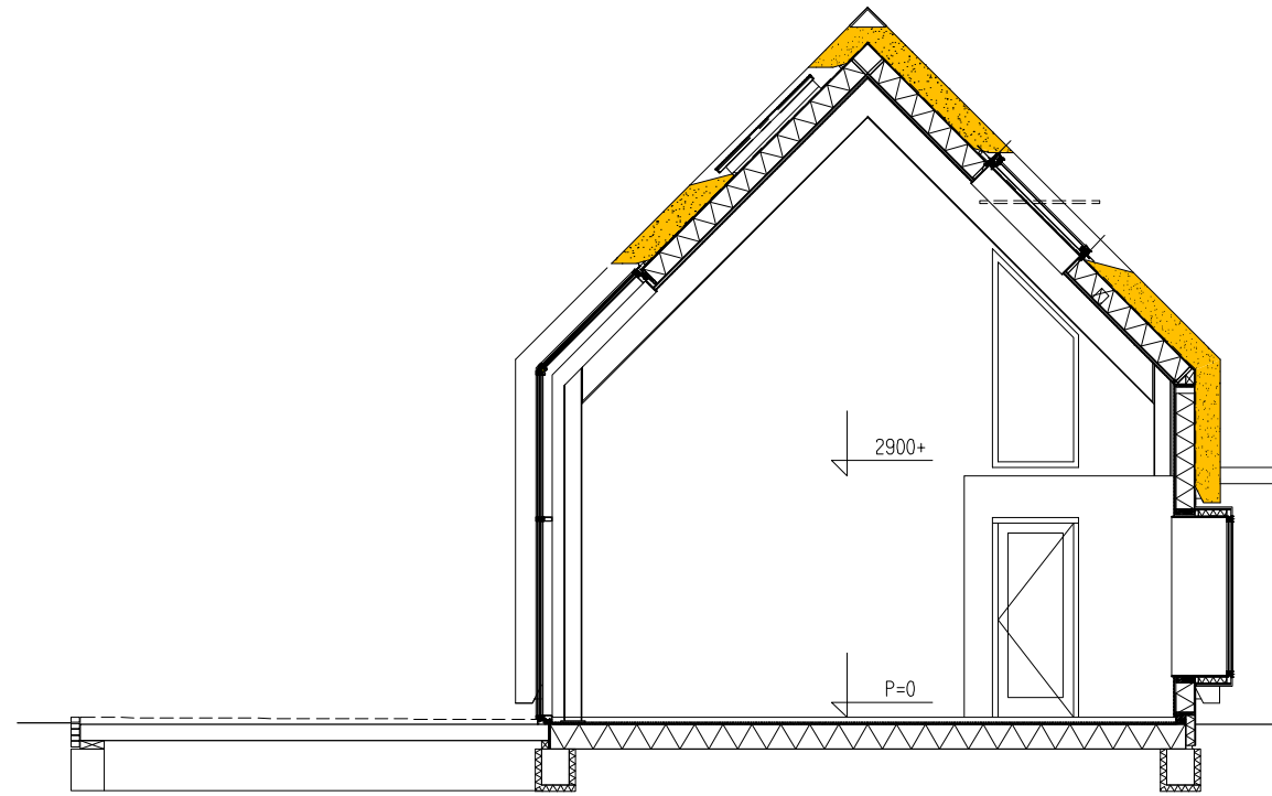
PRINCIPE DOORSNEDE 1
